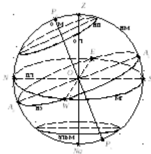
Рис. 1.1. Основные элементы небесной сферы
